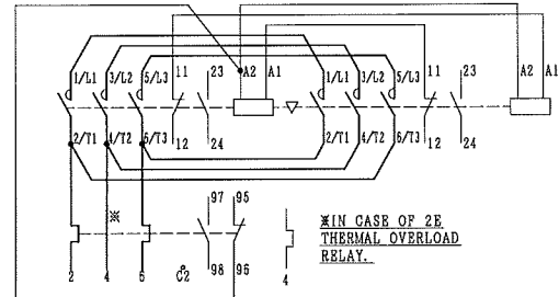
AUX. CONTACTS: 1a1b x 2 CONTACTS ARRANGEMENT.
