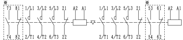
AUX. CONTACTS : 1 b CONTACTS ARRANGEMENT.
