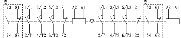
AUX. CONTACTS : 1 b CONTACTS ARRANGEMENT.
