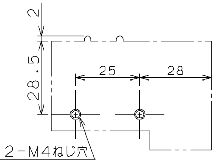
せん孔図
