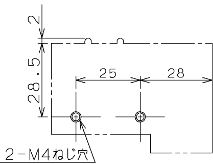
せん孔図
